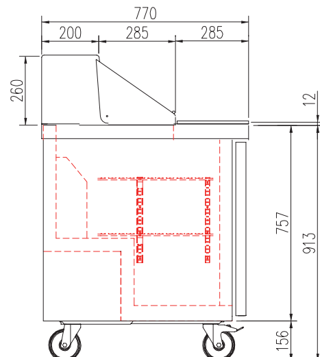
SDT-72 con cajonera opcional with optional drawer set
