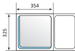
GN 2/3 325 X 354
