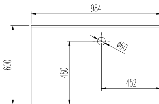
VISTA TALADRO ENCIMERA
