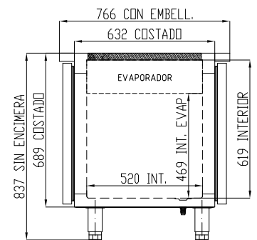
SECCIÓN SIN ENCIMERA
