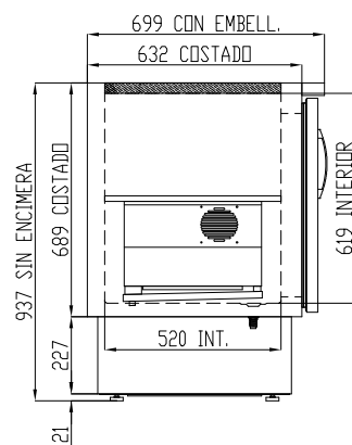
SECCIÓN SIN ENCIMERA
