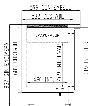
SECCIÓN SIN ENCIMERA
