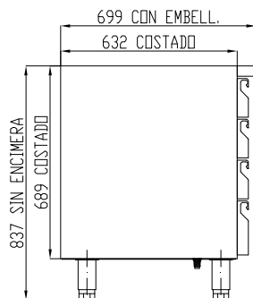
MÓDULO 4 CAJONES
