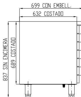
MÓDULO 7 CAJONES
