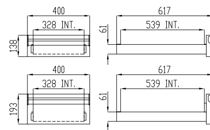
MÓDULO 4 CAJONES
