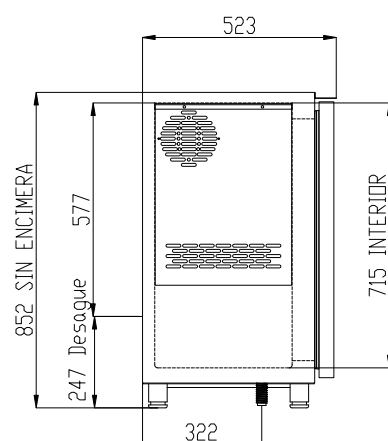
SECCIÓN SIN ENCIMERA
