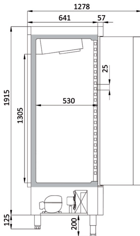
ACRV-125-2
