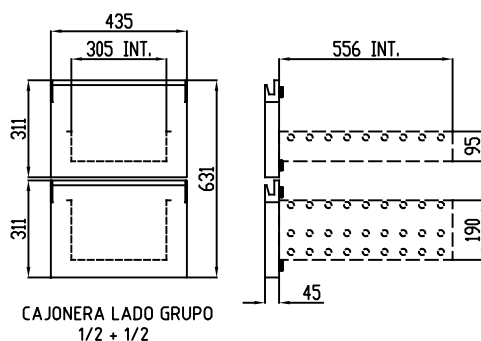
CAJÓN GASTRO 1/2 (LADO GRUPO)
