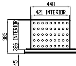
CAJÓN INFERIOR
