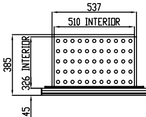
CAJÓN INFERIOR
