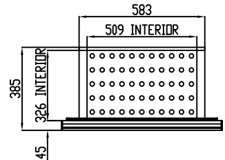
CAJÓN INFERIOR
