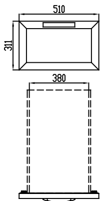
CAJÓN PASTELERA 1/2 (LADO GRUPO)
