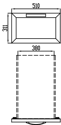
CAJÓN PASTELERA 1/2
