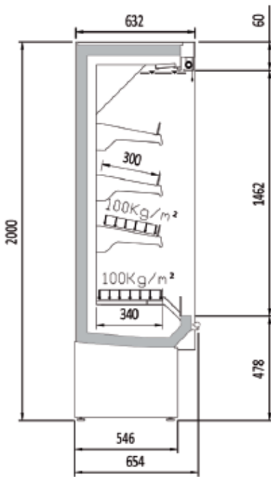
CDS0 H1
