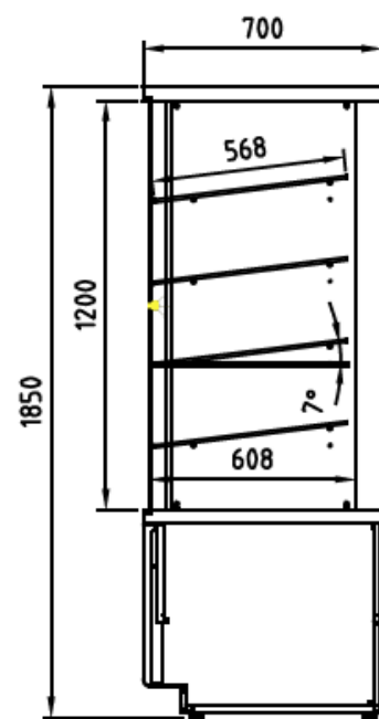
SECCIÓN CMCT-70-RC
