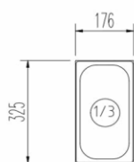
CUBETA G.N.1/3 prof.150mm COD-604.1090009
