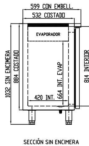
SECCIÓN SIN ENCIMERA
