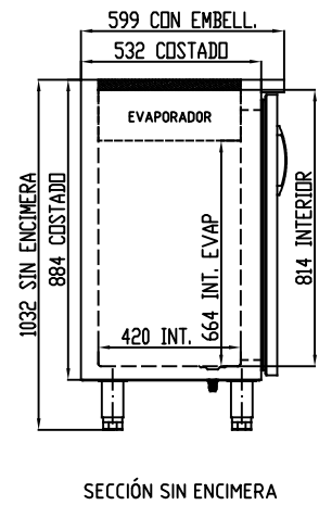
SECCIÓN SIN ENCIMERA
