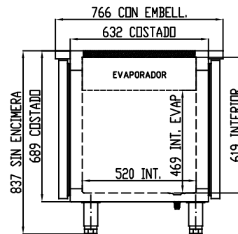
SECCIÓN SIN ENCIMERA
