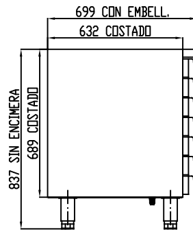
MÓDULO 7 CAJONES
