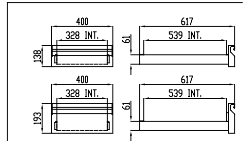
MÓDULO 4 CAJONES
