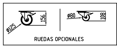
ALTURA MÍN. Y MAX. PATA OPCIONAL
