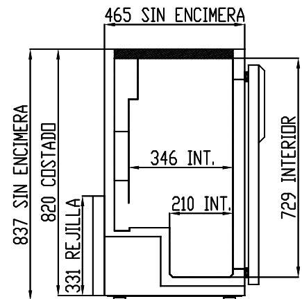
SECCIÓN SIN ENCIMERA
