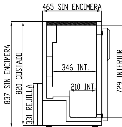
SECCIÓN SIN ENCIMERA
