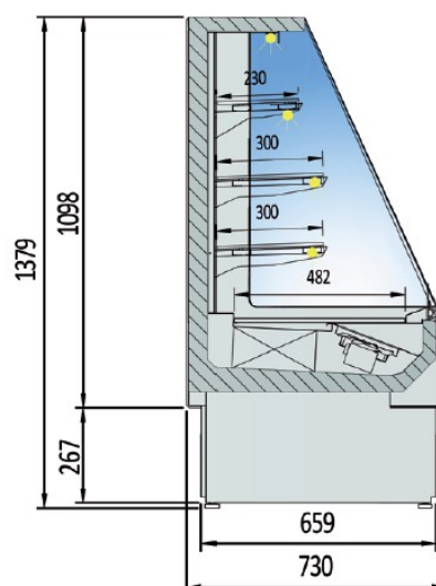
VSSAM-6
