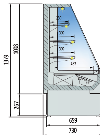
VSSAM-6
