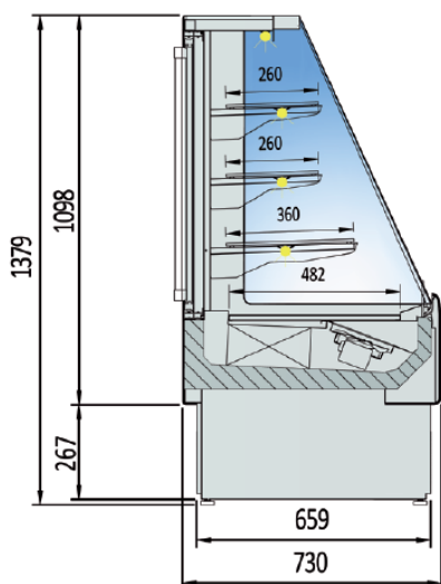
VSS / VSSA-6
